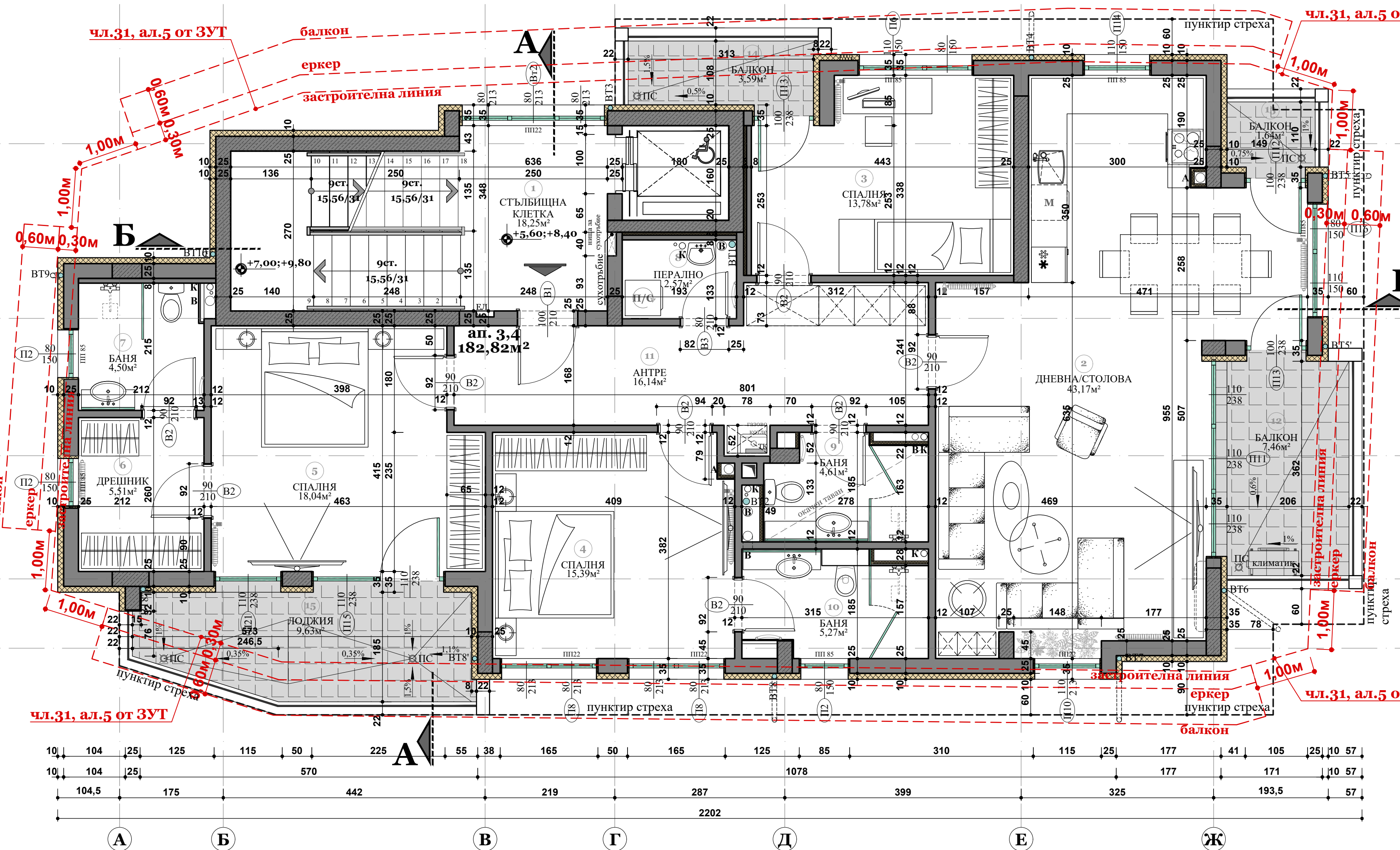
РАЗПРЕДЕЛЕНИЕ ТИПОВ ЕТАЖ МАЩАБ 1:50
