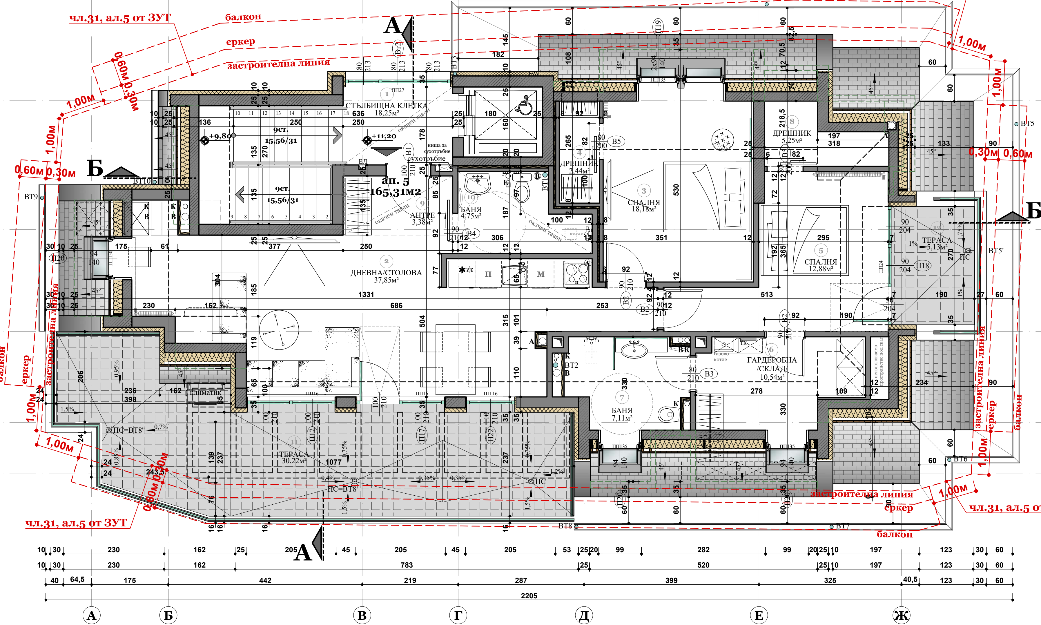
РАЗПРЕДЕЛЕНИЕ МАНСАРДЕН ЕТАЖ МАЩАБ 1:50
