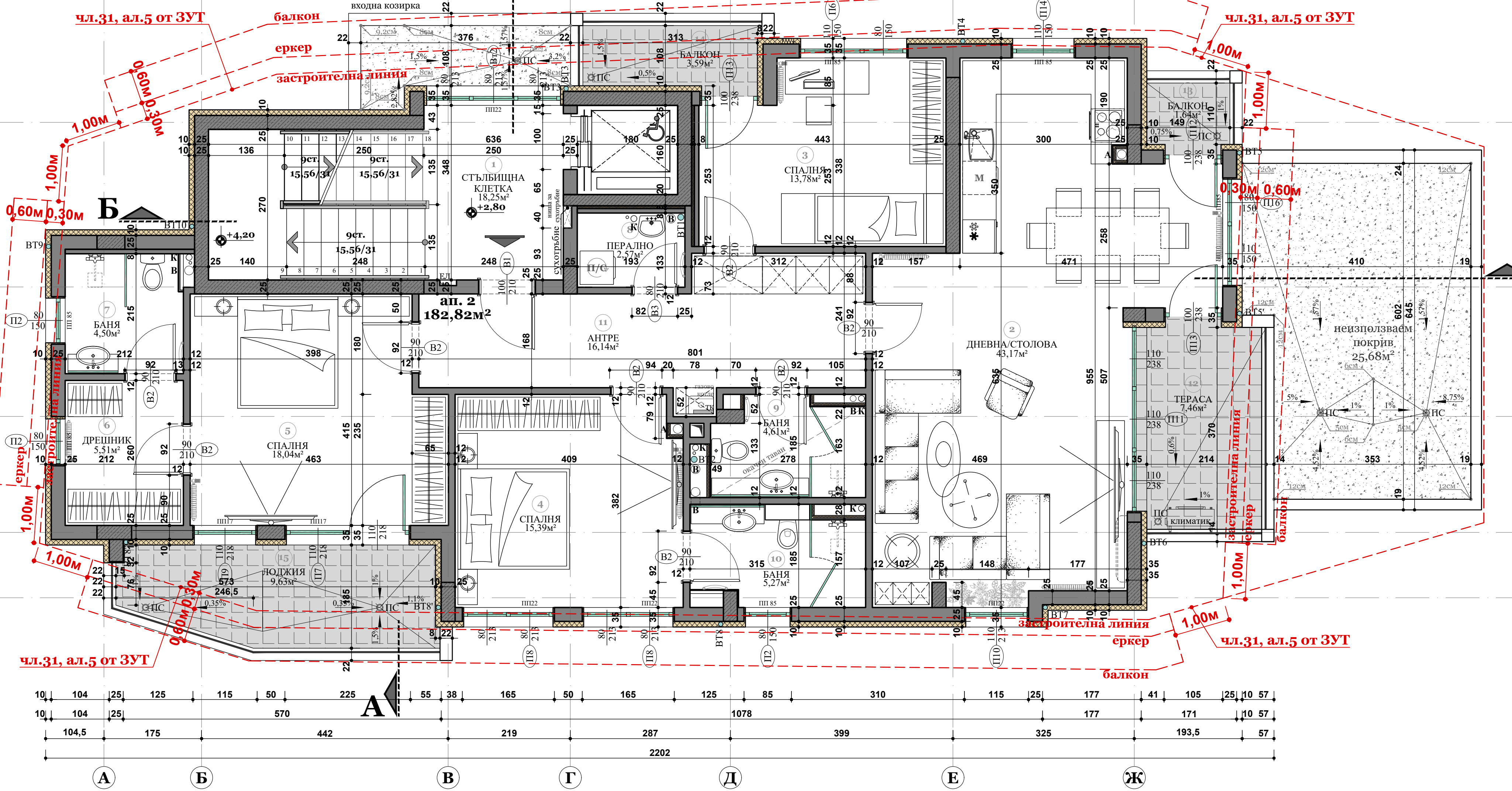
РАЗПРЕДЕЛЕНИЕ ВТОРИ ЕТАЖ МАЩАБ 1:50
