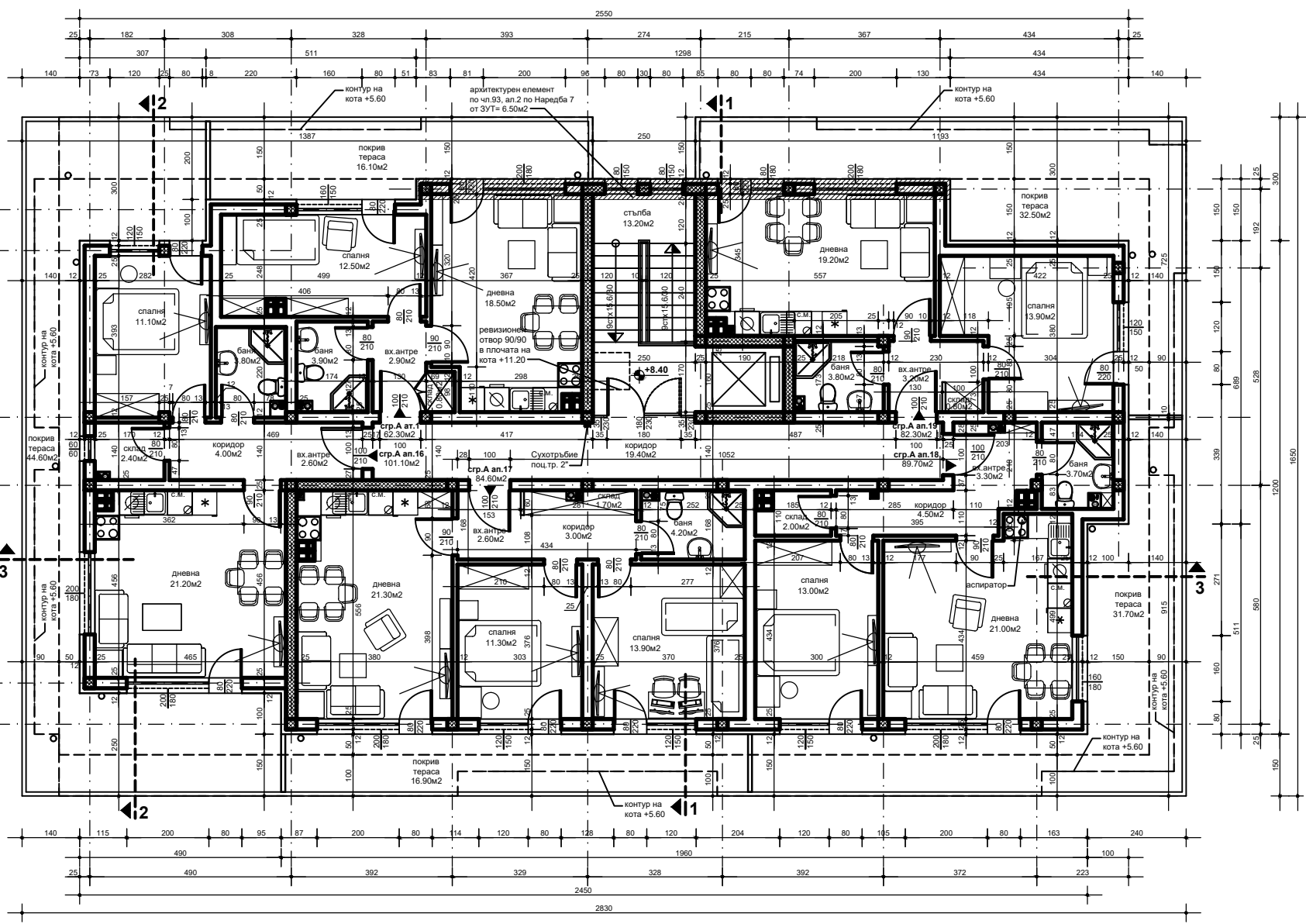
РАЗПРЕДЕЛЕНИЕ МАНСАРДЕН ЕТАЖ - КОТА +8.40 М 1 : 50
