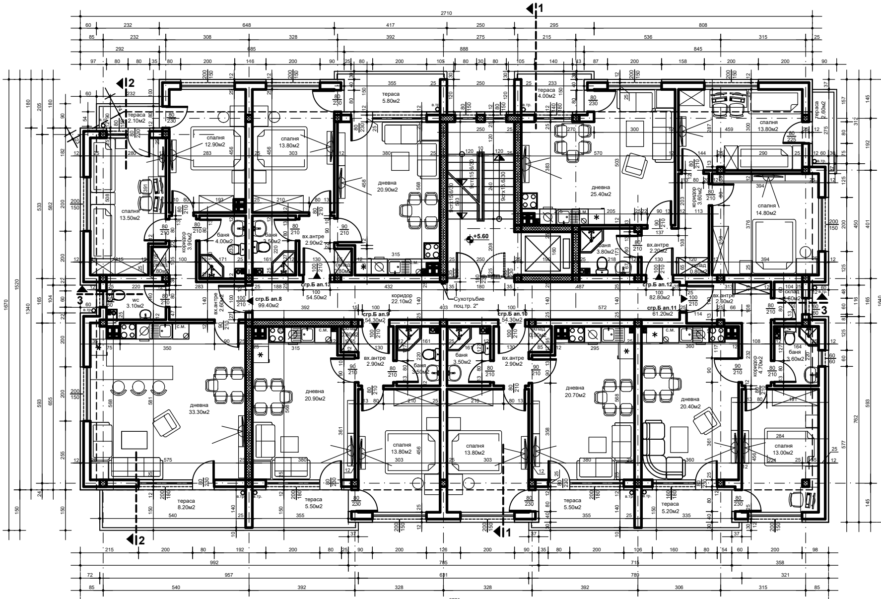
РАЗПРЕДЕЛЕНИЕ ТРЕТИ ЕТАЖ - КОТА +5.60 M 1 : 50
