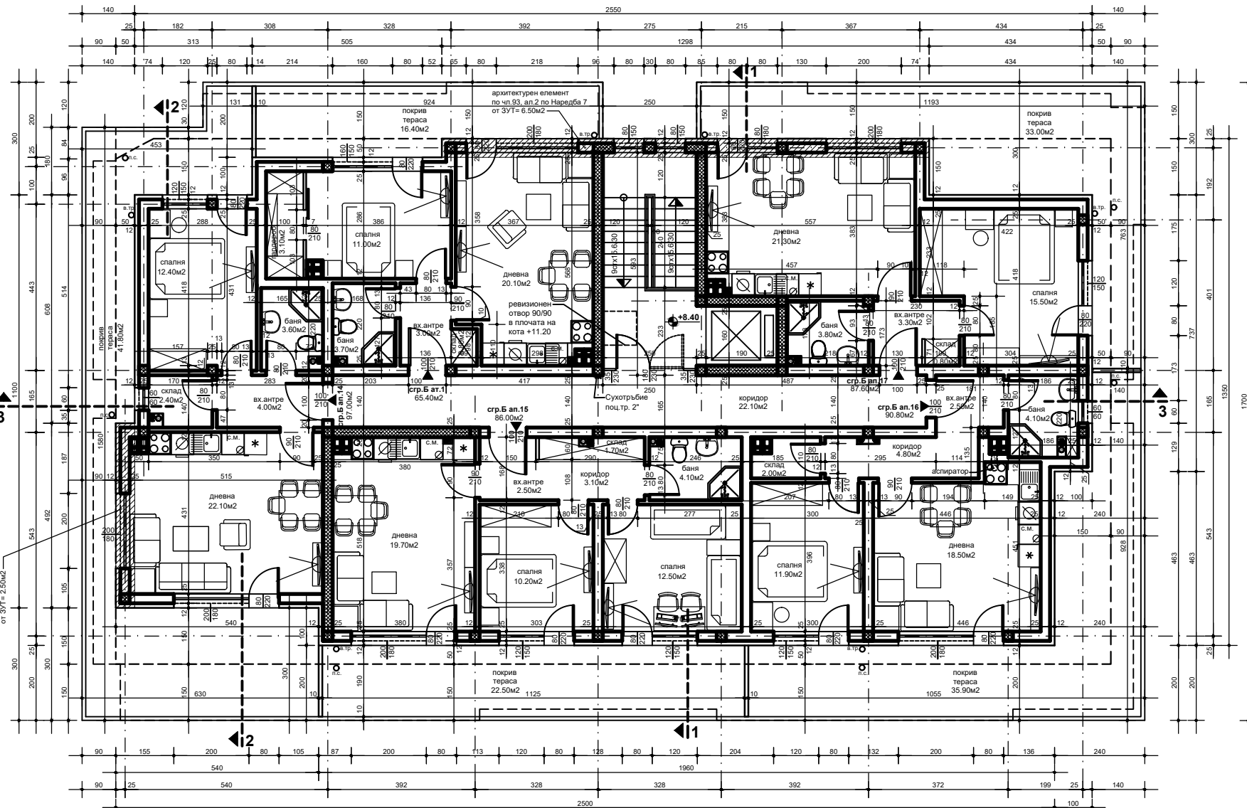
РАЗПРЕДЕЛЕНИЕ МАНСАРДЕН ЕТАЖ - КОТА +8.40 М 1 : 50
