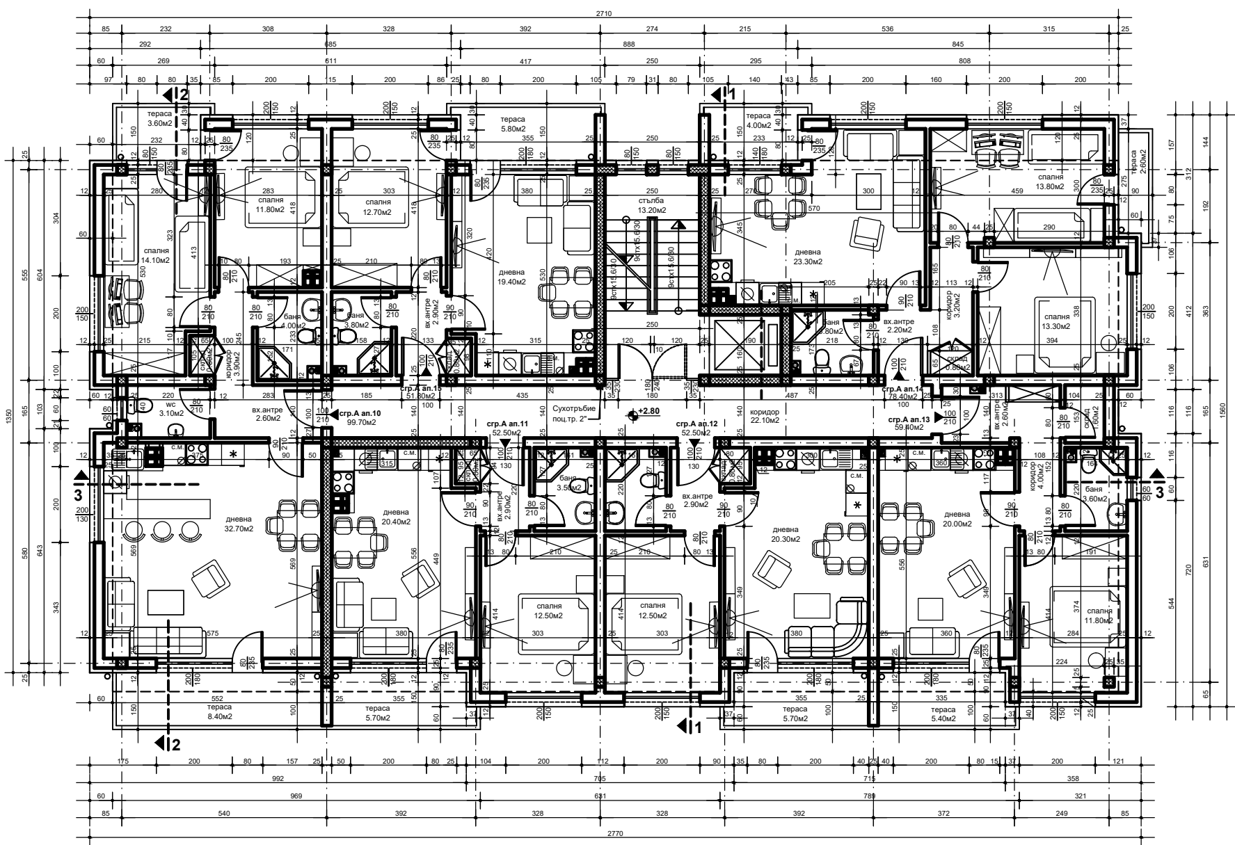
РАЗПРЕДЕЛЕНИЕ ТРЕТИ ЕТАЖ - КОТА +5.60
