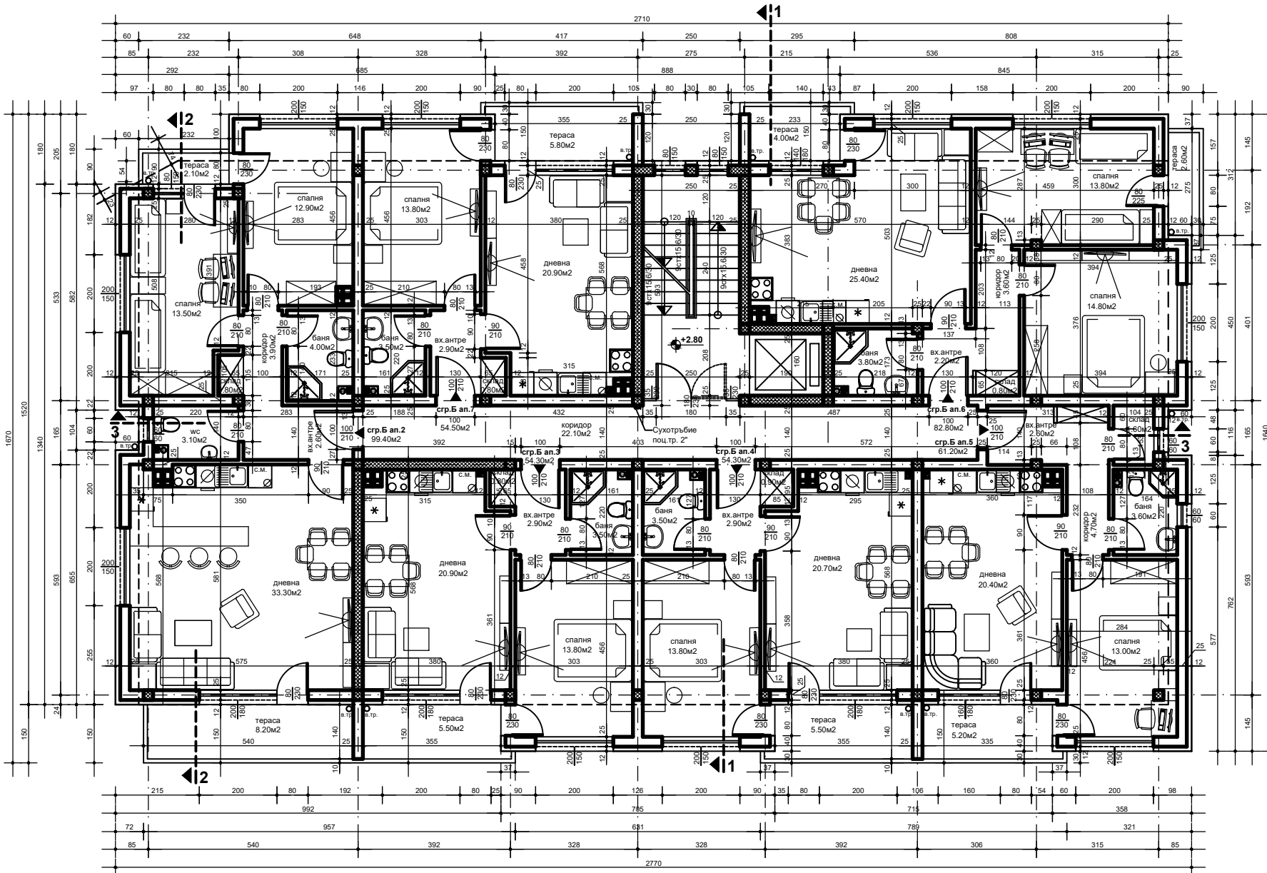
РАЗПРЕДЕЛЕНИЕ ВТОРИ ЕТАЖ - КОТА +2.80 М 1 : 50
