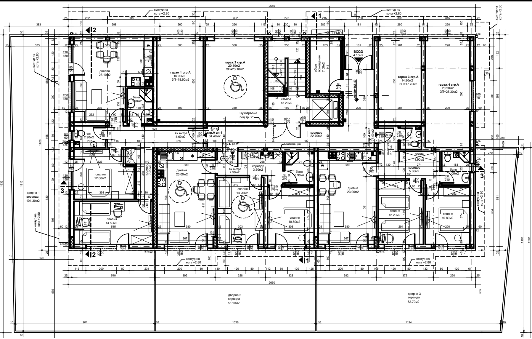
ЖИЛИЩНА СГРАДА А - РАЗПРЕДЕЛЕНИЕ ПЪРВИ ЕТАЖ (ПАРТЕР)
