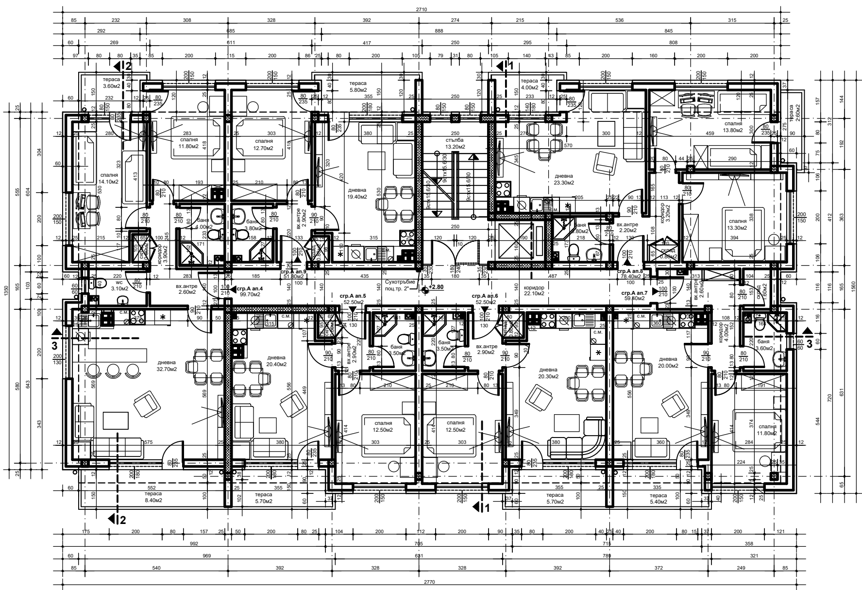
РАЗПРЕДЕЛЕНИЕ ВТОРИ ЕТАЖ - КОТА +2.80
